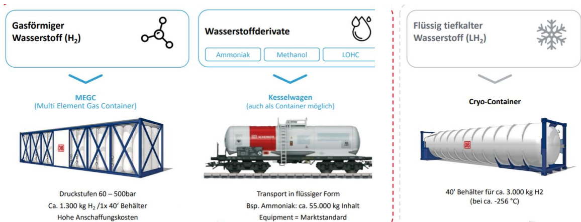
Abbildung 3-20: Formen des schienenengebundenen Wasserstofftransports (35)
