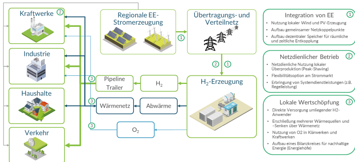
Abbildung 2-9: H 2 -Wertschöpfungskette in integrierter Energieversorgung (eigene Darstellung)
